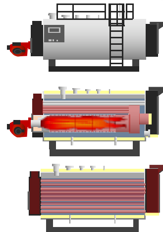
ESQUEMA SECCIÓN CALDERA
